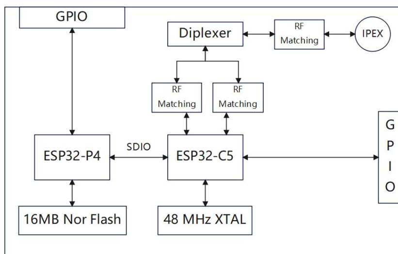
图5: WT01P4C5-S1 硬件框图
