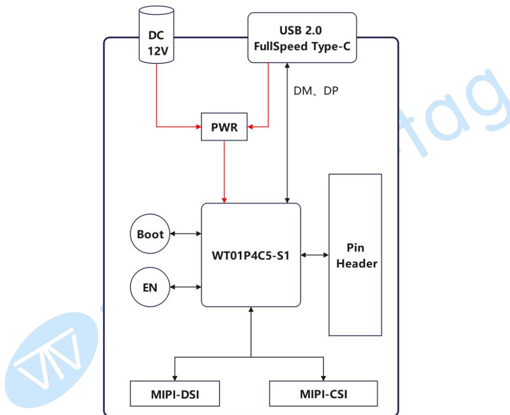
图4: WTDKP4C5-S1 功能框图
