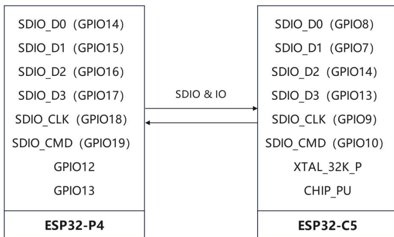
图6: P4 & C5 引脚对应图
