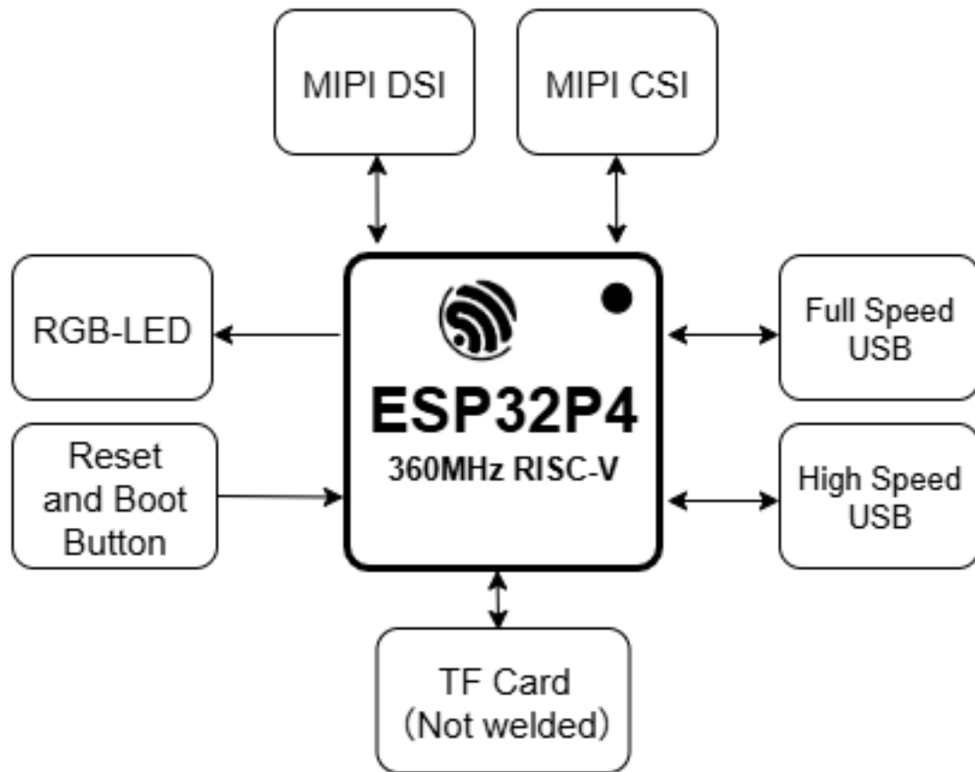
图 1 - 功能框图
