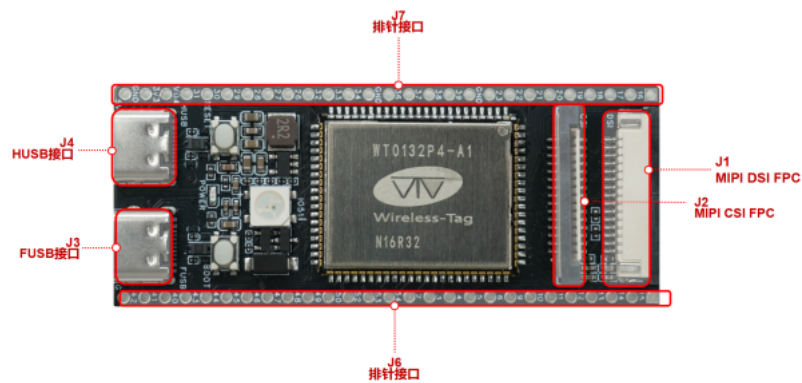
图 2 – 正面接口组件
