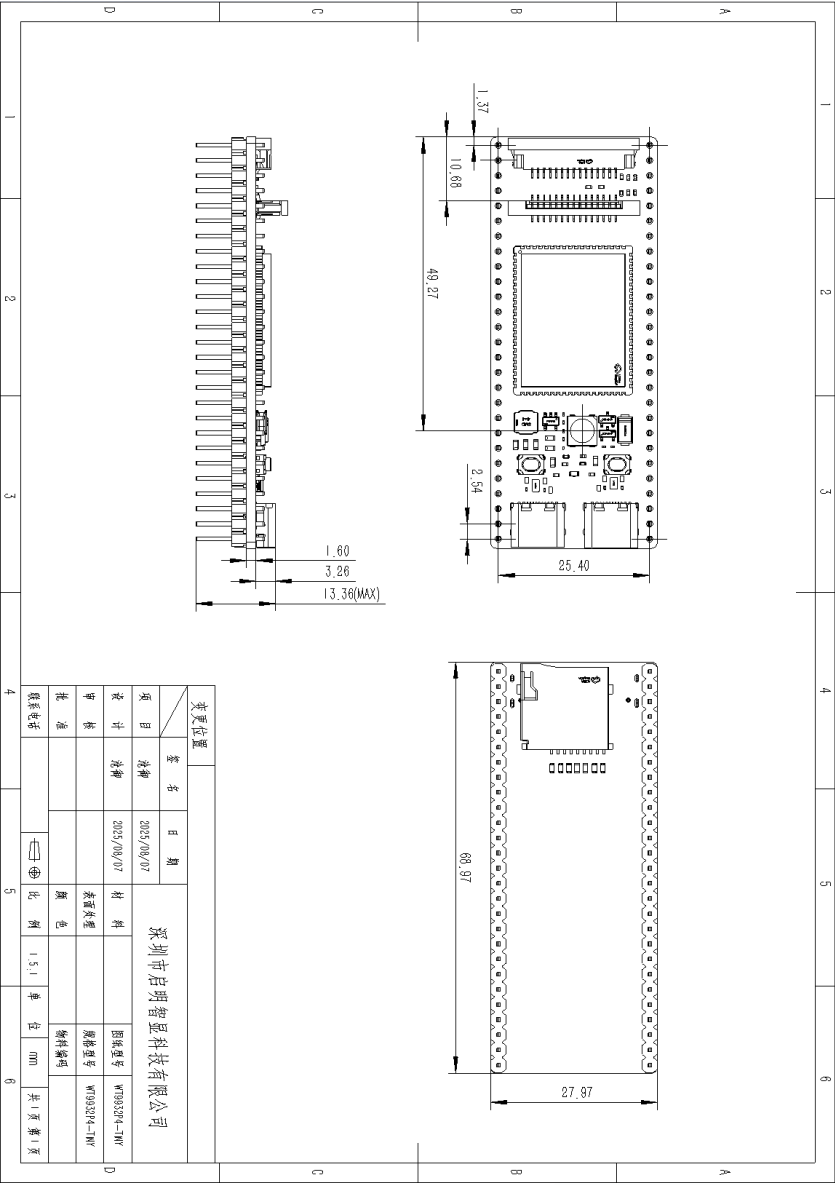
图 6 - 主板尺寸图
