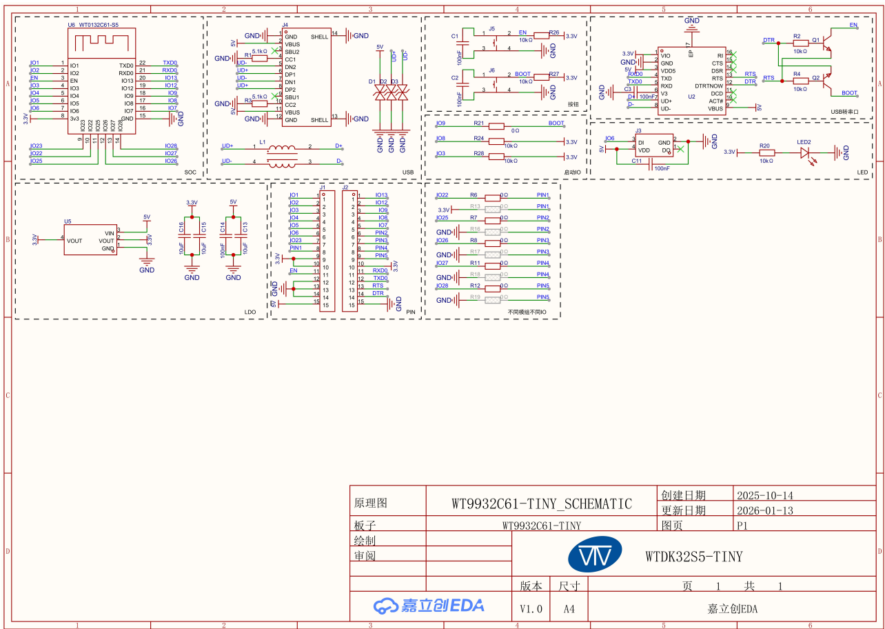
图 5 - 原理图
