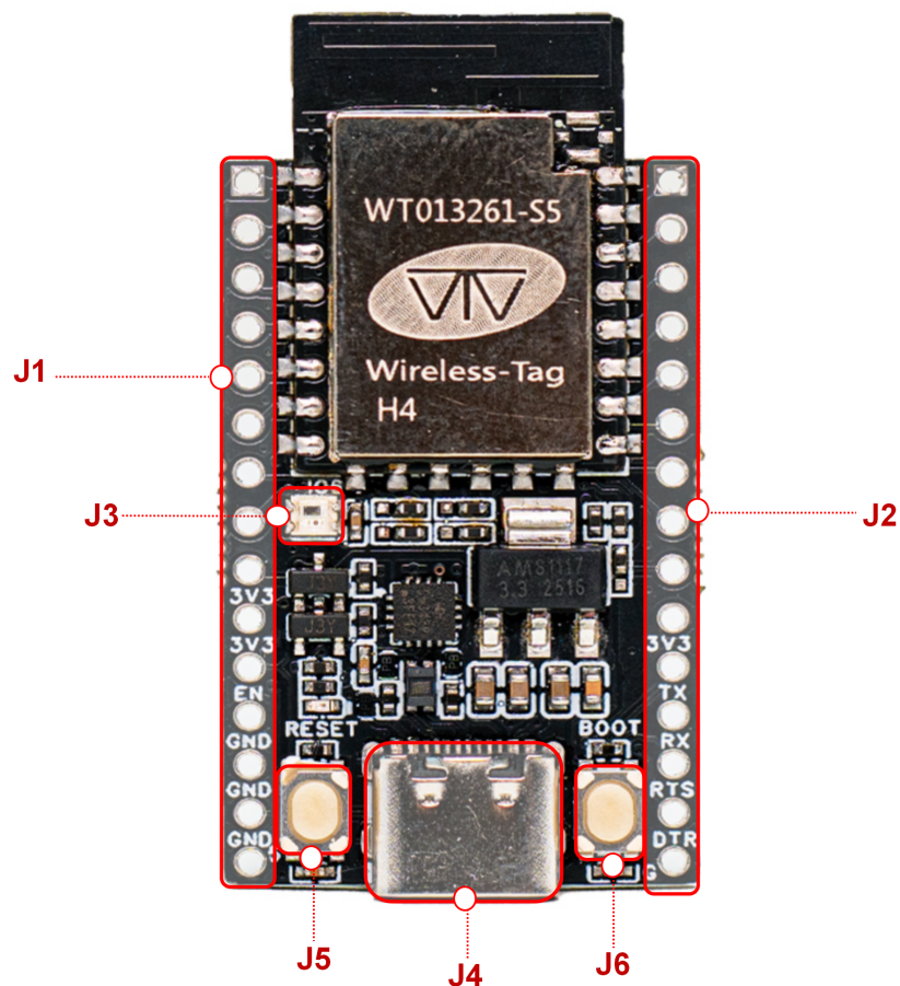
图 4 - 接口组件
