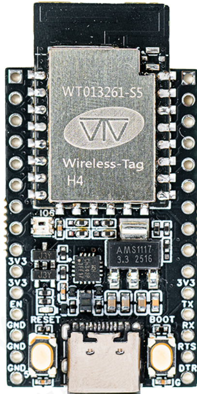
图 1 - 开发板图片
