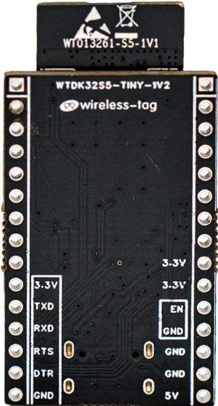
图 2 - 开发板图片
