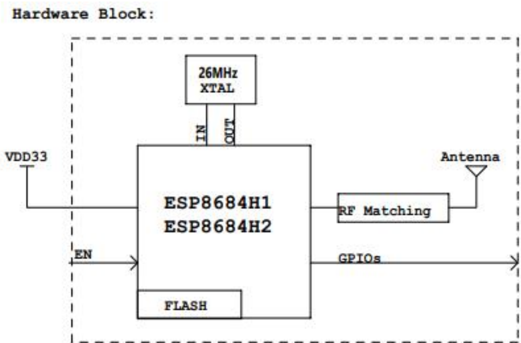
图 1 硬件框图
